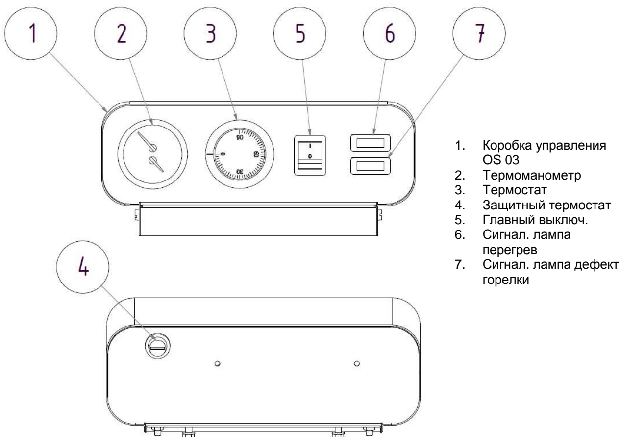
Рис. 13 Коробка управления OS 03
